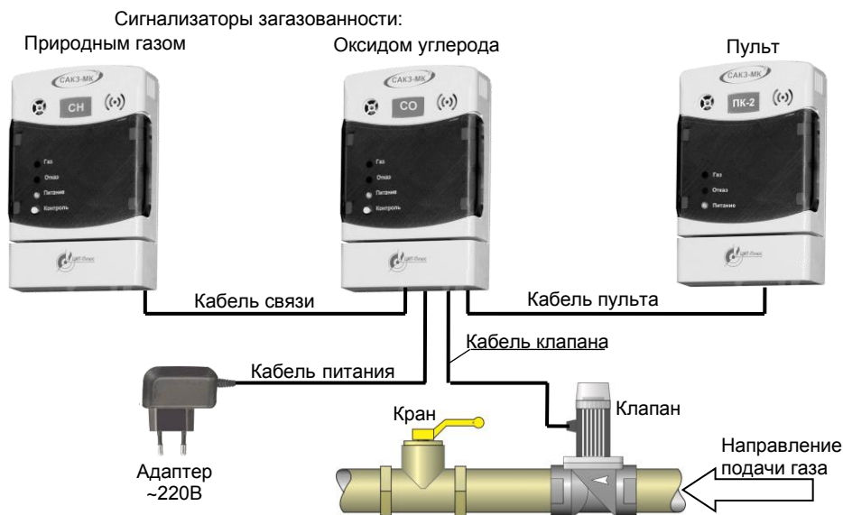
Рисунок 1 - Структурно-функциональная схема стандартной системы
