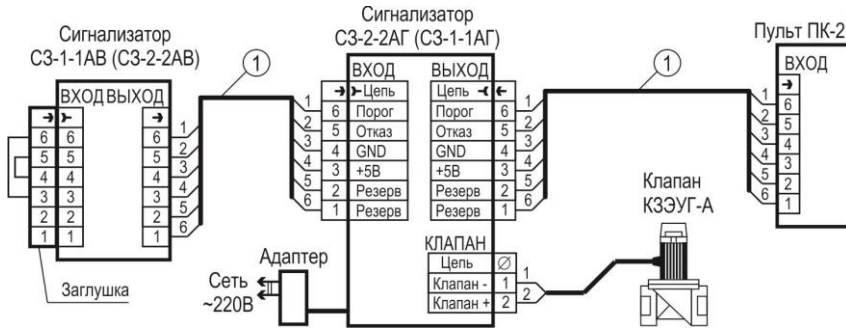
Рисунок Б.1 – Типовая схема соединений
