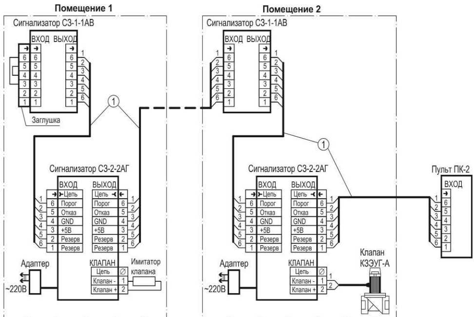
Рисунок Б.1 – Типовая схема соединений
