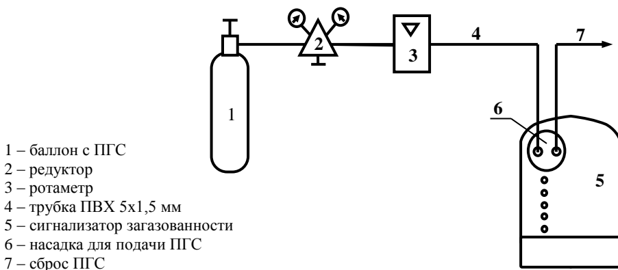
Рисунок Ж.2 – Схема для настройки порога срабатывания и проверки сигнализатора с применением ПГС
